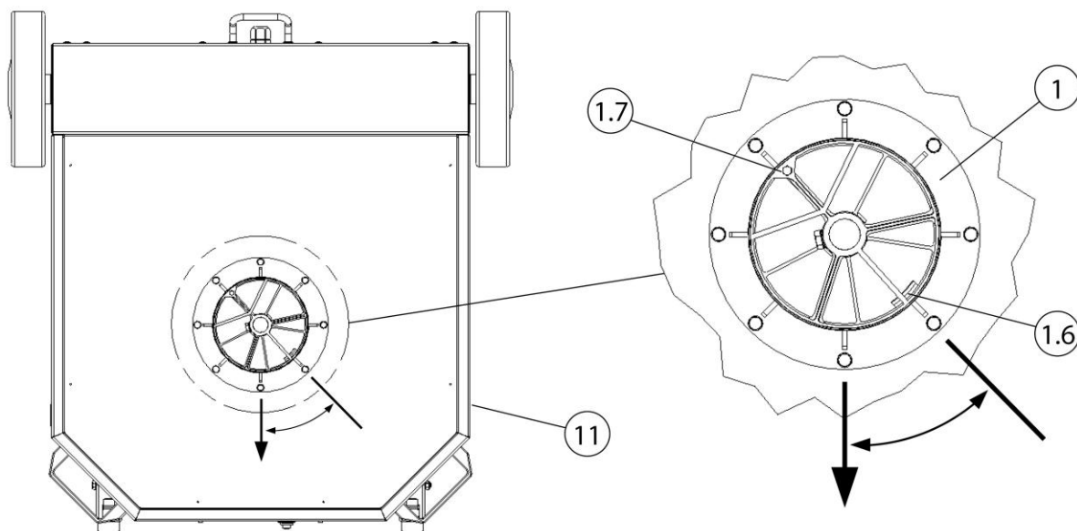
8. ábra: A forgókoszorú kiszintezése
