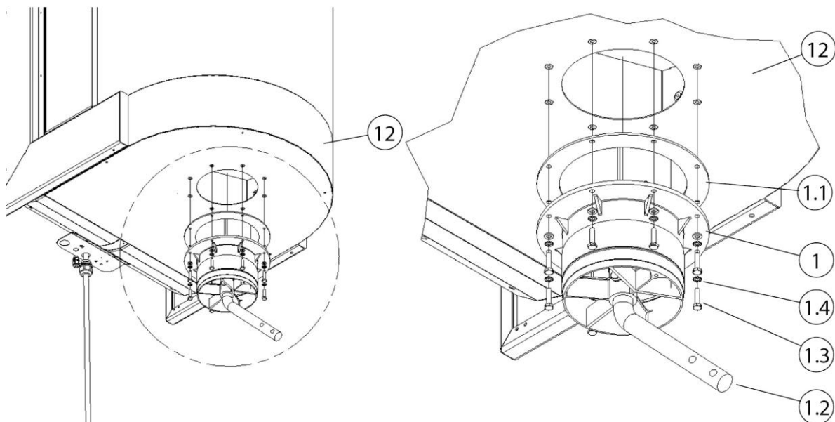
10. ábra: Helyhez kötött szűrőkészülék összeszerelése
