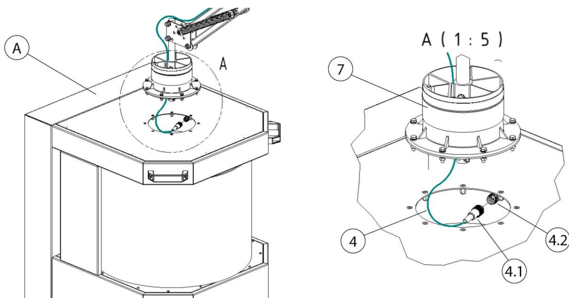
18. ábra: Csatlakoztatás - Mobil szűrőkészülék
