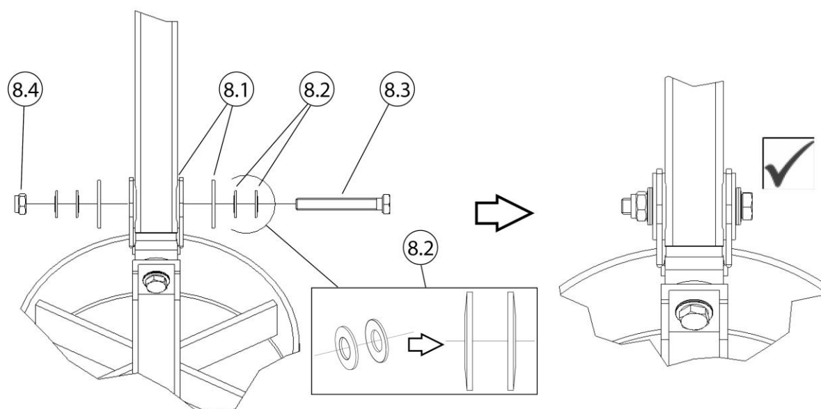
16. ábra: A szívóbúra felszerelése
