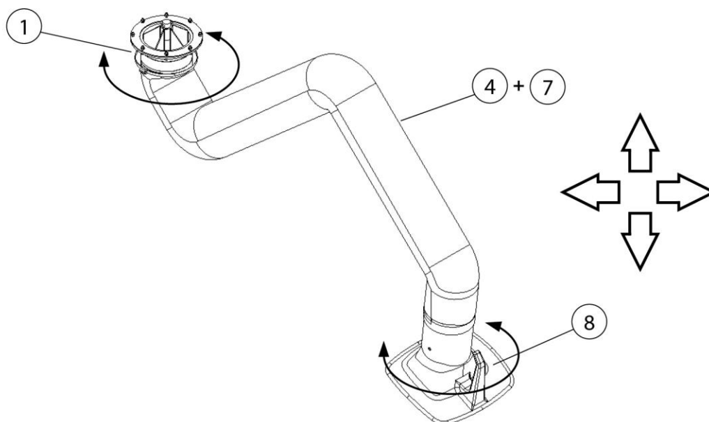
1. ábra: Szívókar - Működési leírás
